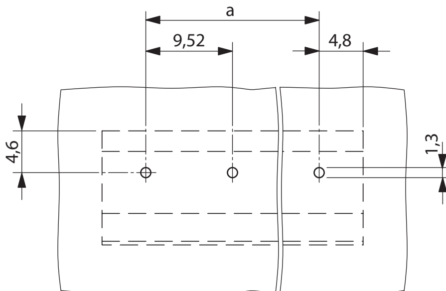
Bohrplan/Lötpadgeometrie
