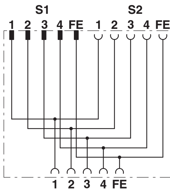
Diagrama eléctrico
