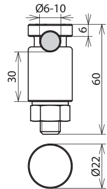
Maßbild KSVL 6.10 FER V2A
