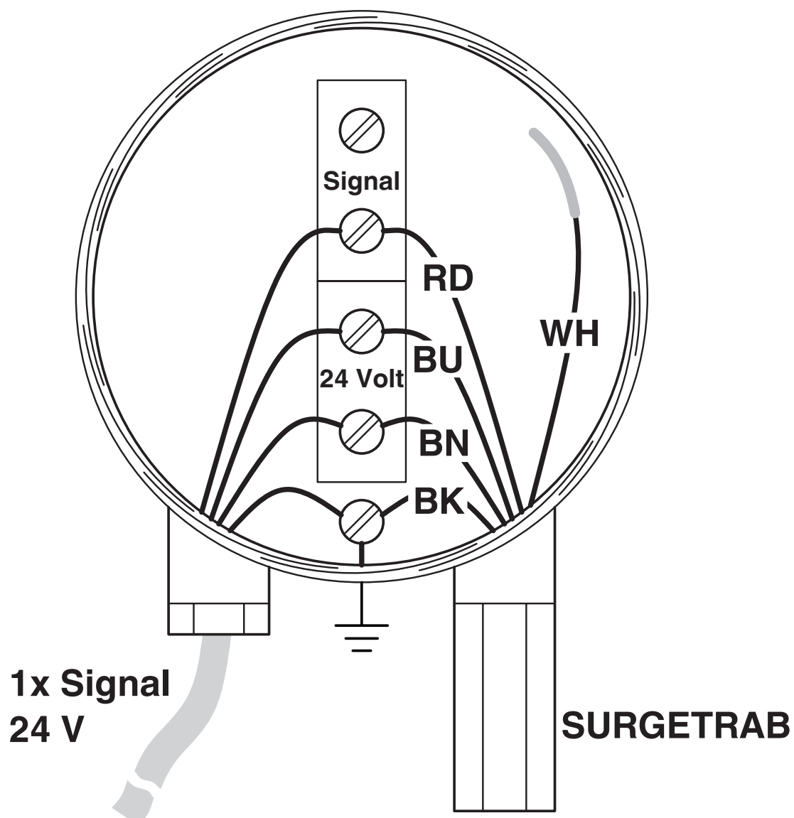
Applikationszeichnung
