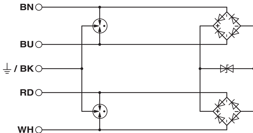
Schaltplan
