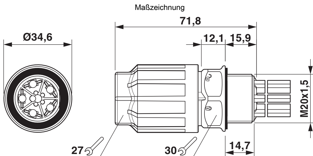
Maßzeichnung des QPD W 5x2,5 M20
