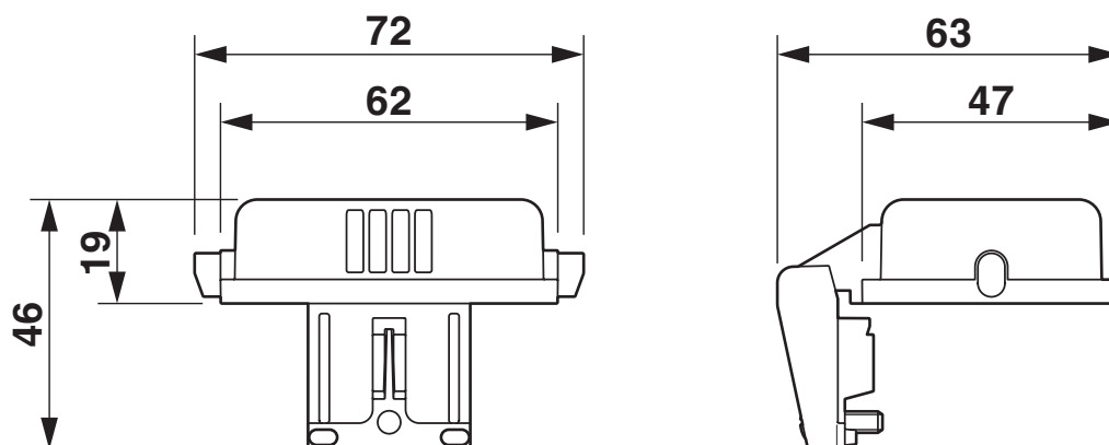
Dessin coté
