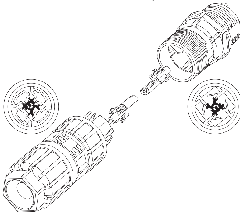
Schemazeichnung
