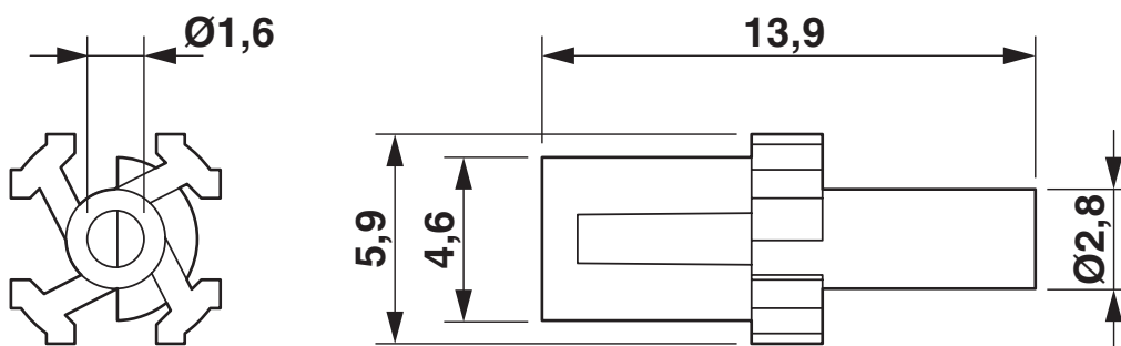
Maßzeichnung
