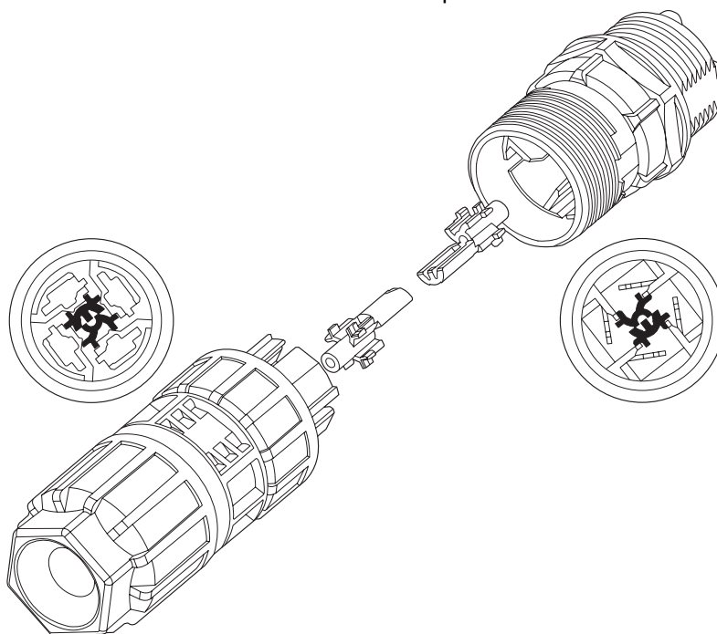
Dessin schématique
