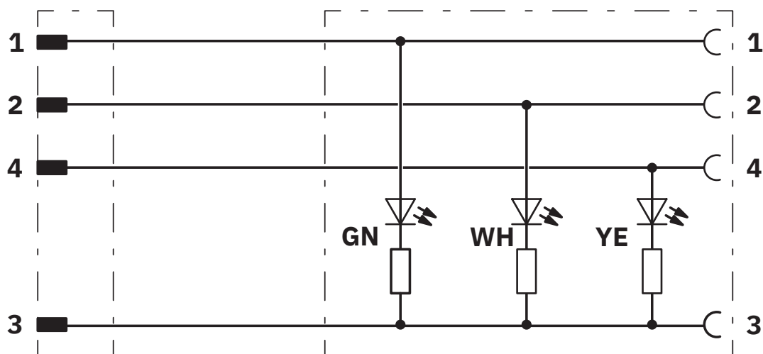
Ocupación de contactos del conector macho M12 y del conector hembra M12
