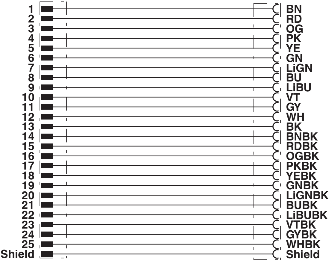
Diagrama eléctrico
