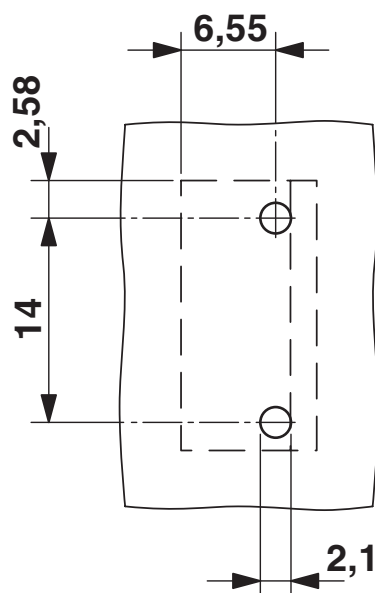
Gabarit perçage / géom. pastille soudage
