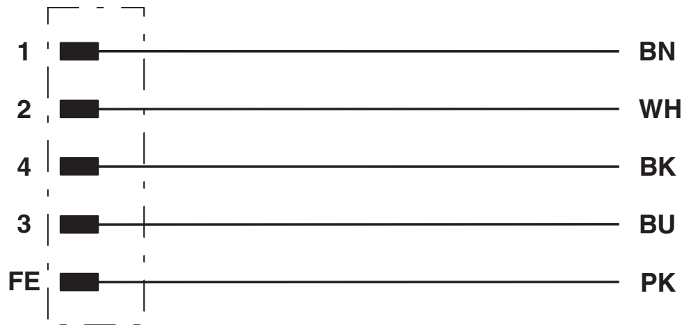
Schaltplan
