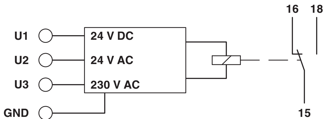
Schéma fonctionnel
