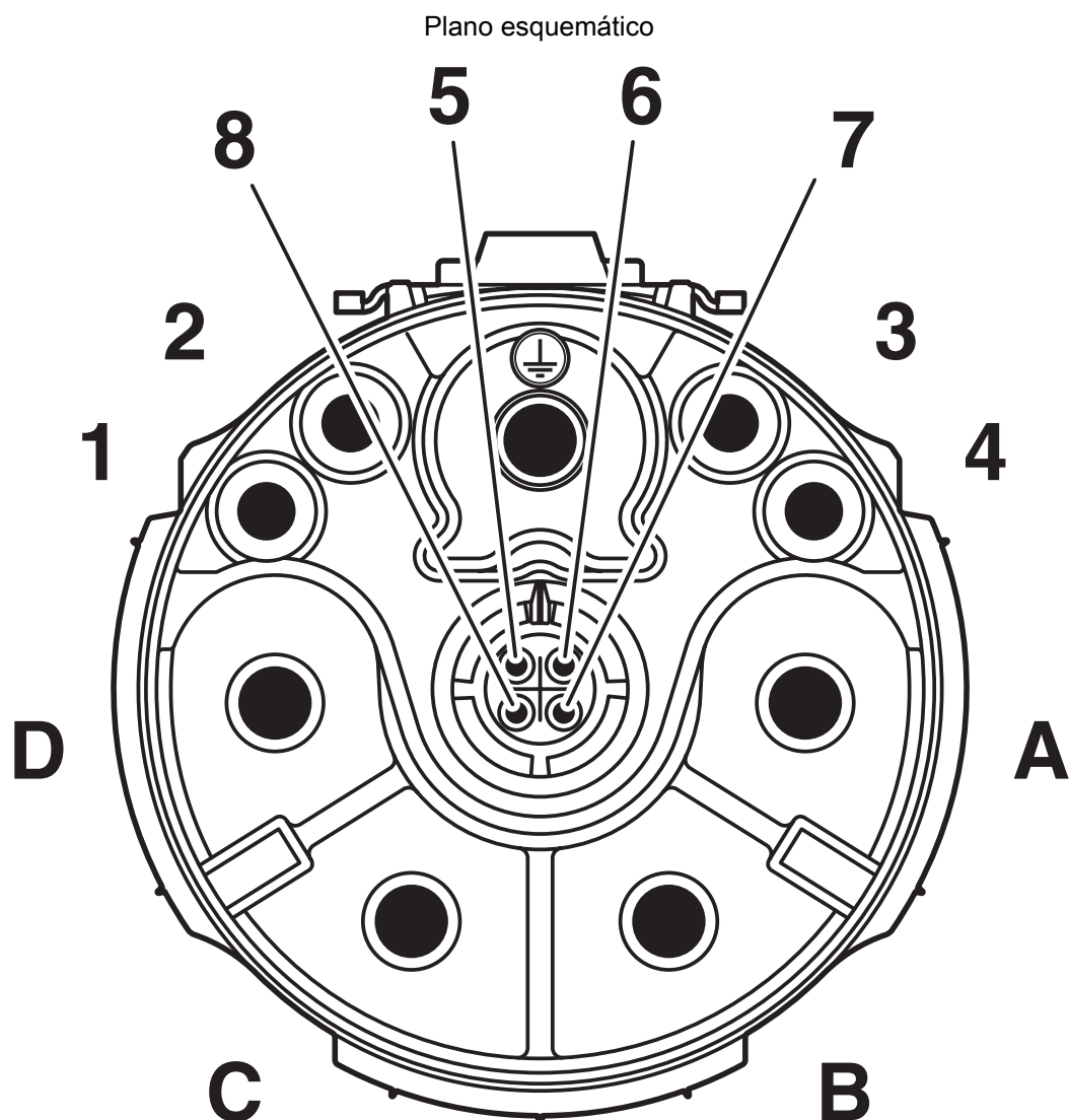
Esquema de polos conector macho CAT5, codificación 2
