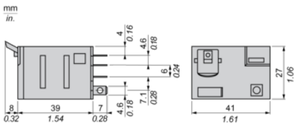
Vista lateral de los pins
