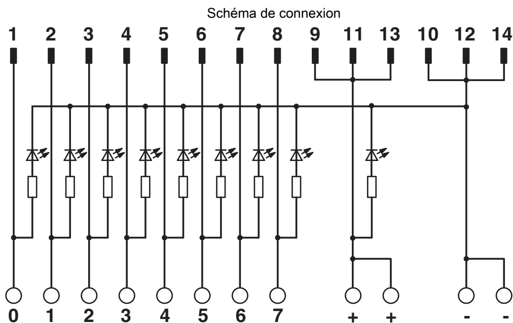
Schéma des connexions VIP-2/.../FLK14/LED/PLC
