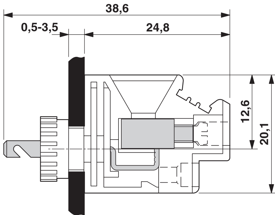
Maßzeichnung
