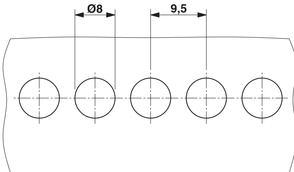
Maßzeichnung
