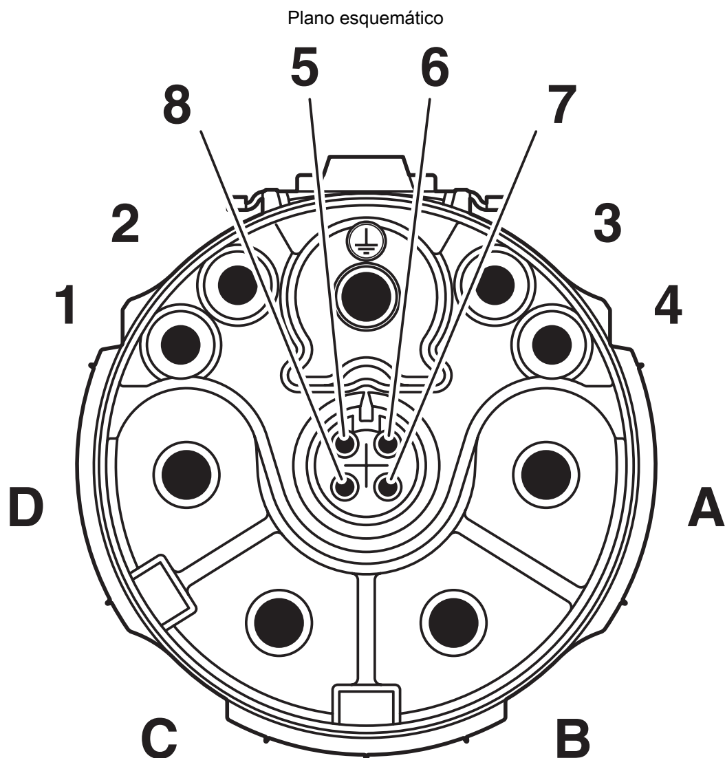
Esquema de polos conector macho señal, codificación 1
