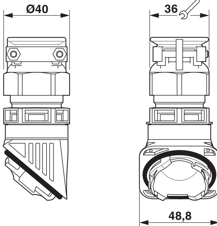
Maßzeichnung
