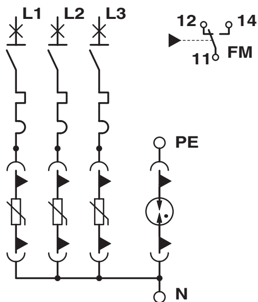
Diagrama eléctrico
