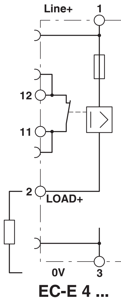
Diagrama eléctrico
