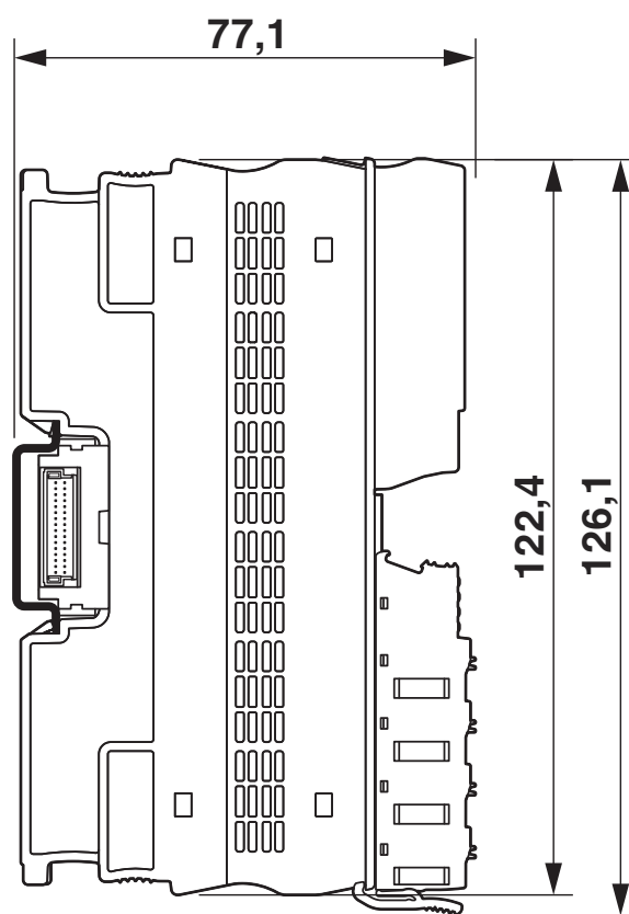
Dessin coté
