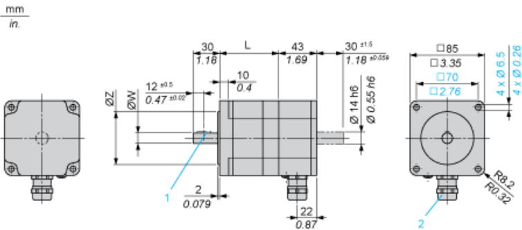
Dimensiones en mm
