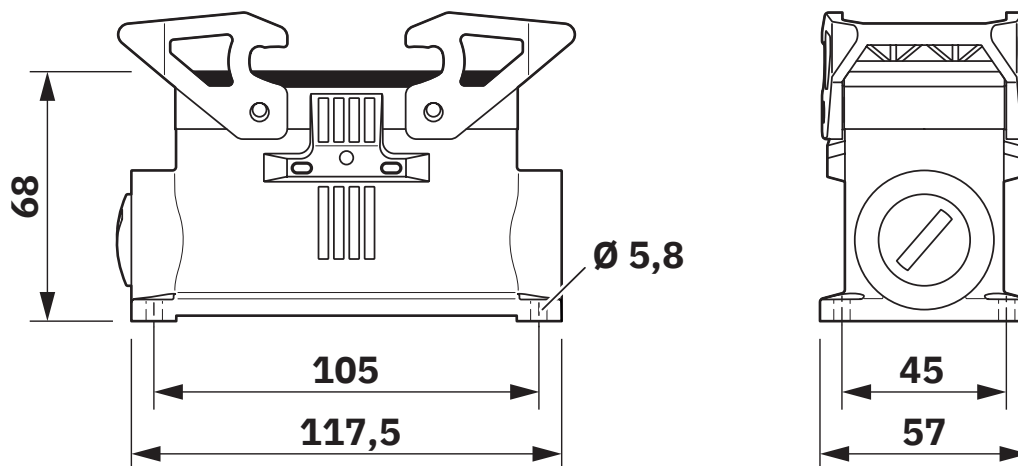
Maßzeichnung
