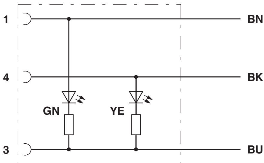
Kontaktbelegung der M8/M12-Buchse mit 2 LED
