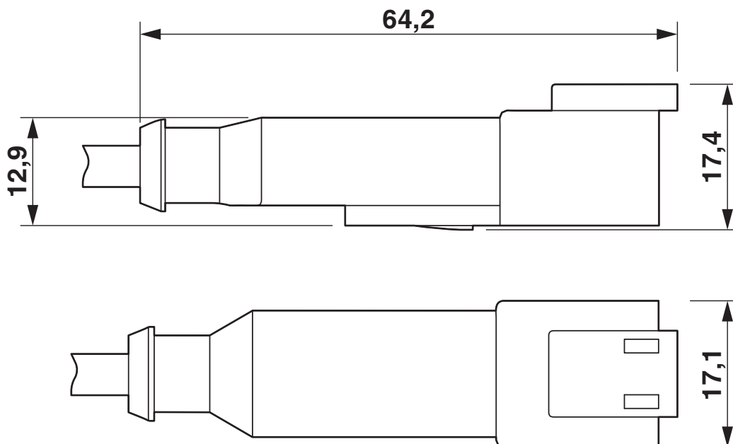
DEUTSCH DT04-2P, Drauf- und Seitenansicht
