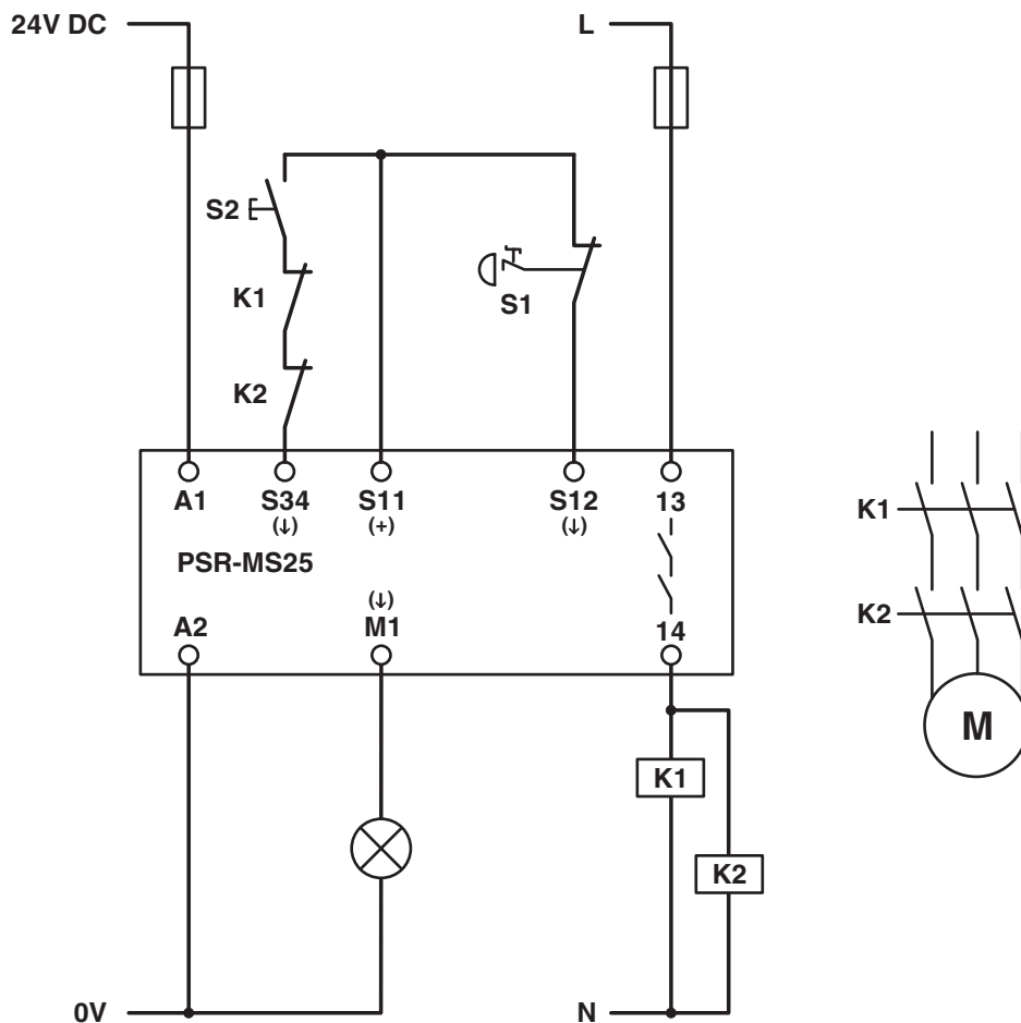
Applikationszeichnung
