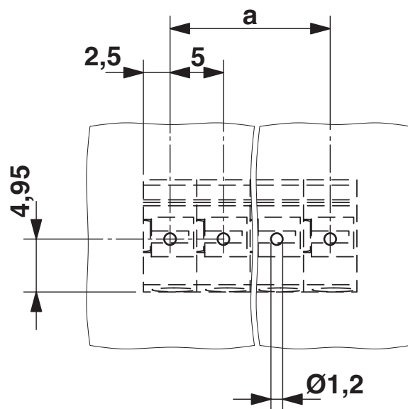
Bohrplan/Lötpadgeometrie
