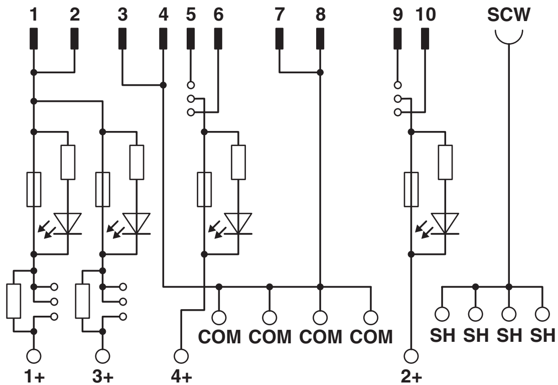
Schaltplan
