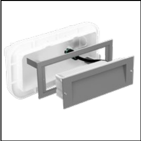
310488 Adaptador INSERT+ 2 (kit reacondicionamiento Insert 2) ■ GR-94 / Gris metalizado
