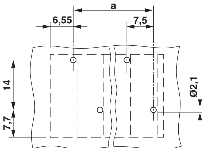
Bohrplan/Lötpadgeometrie
