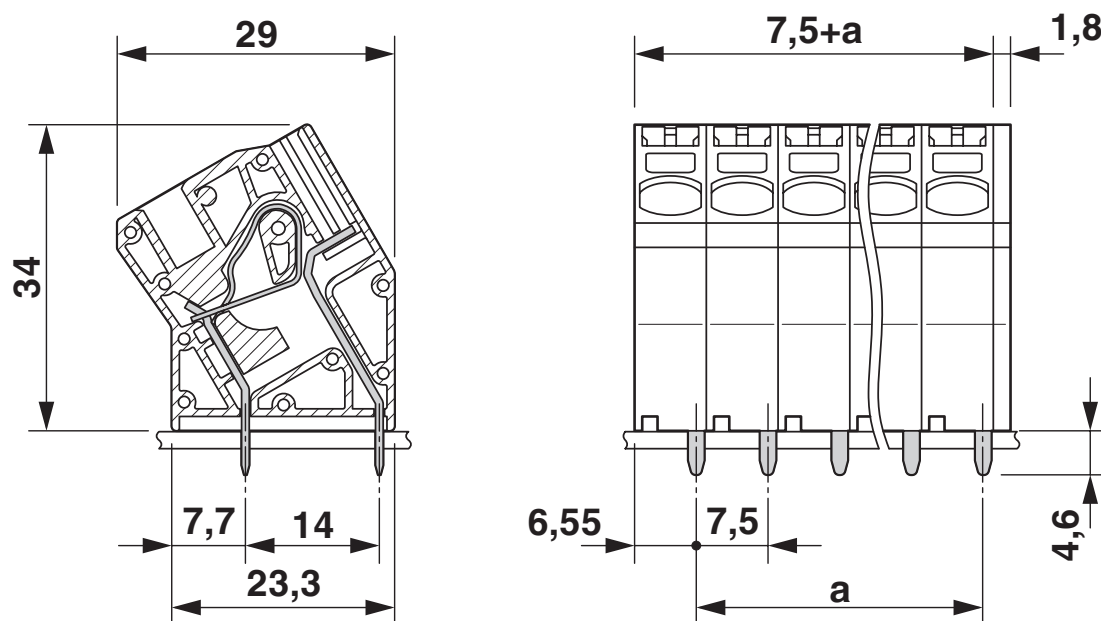
Maßzeichnung
