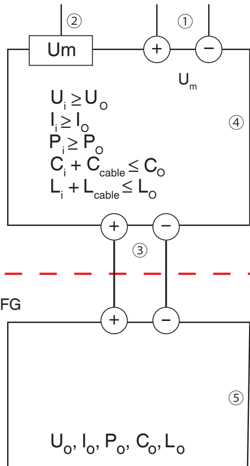
Plano esquemático
