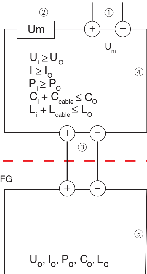
Dessin schématique
