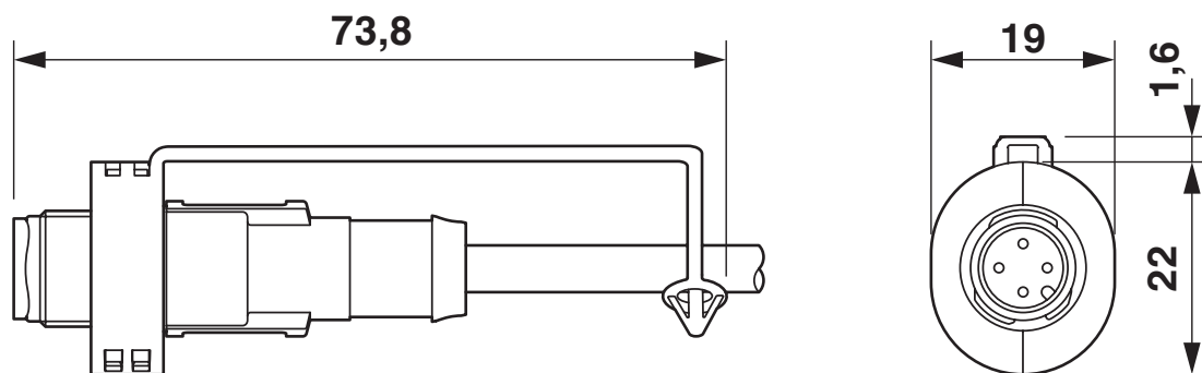
Mit EXCLIP montierter Stecker
