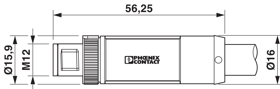
Dessin coté
