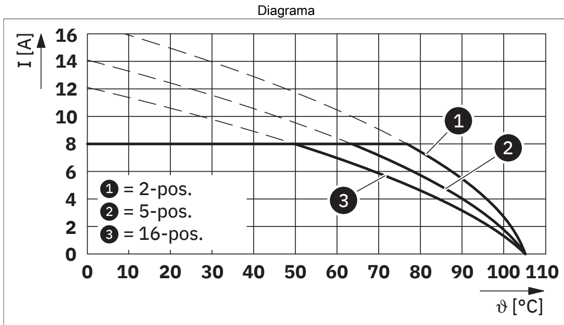
Tipo: FMCOR 1,5/...-ST-3,5 con MC 1,5/...-G-3,5 P... THR
