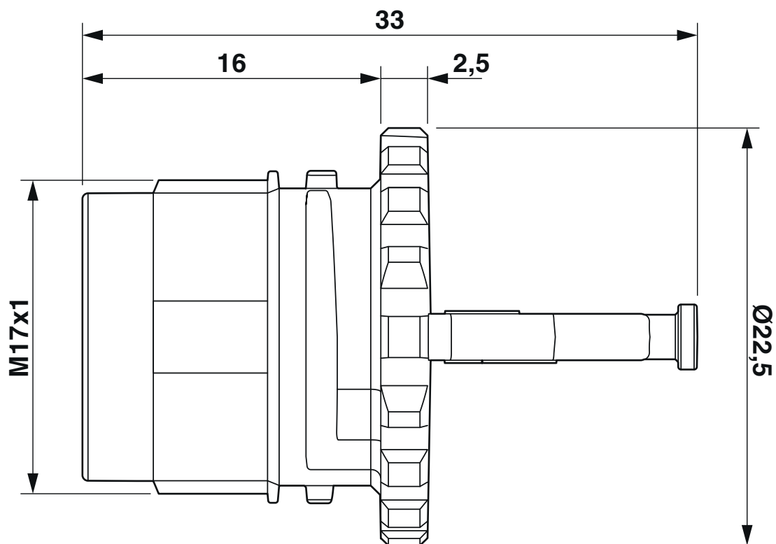
Maßzeichnung
