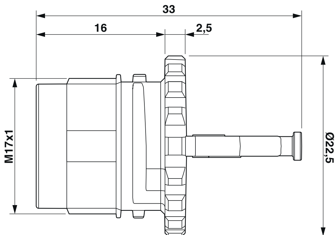
Dessin coté
