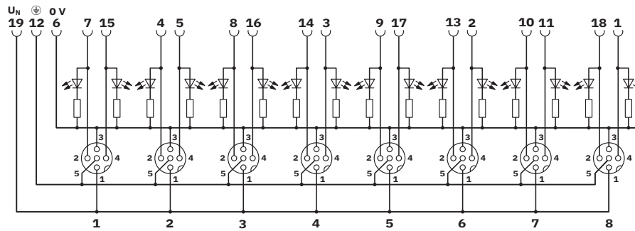
Diagrama eléctrico
