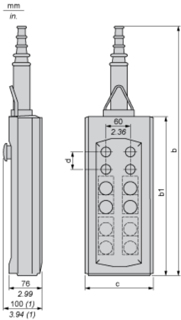
Dimensiones en mm
