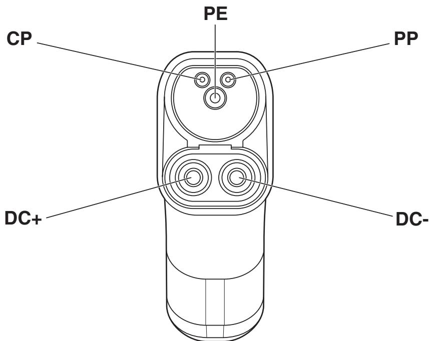
Dessin schématique
