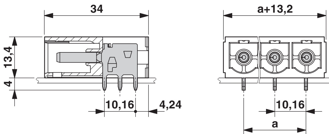
Dessin coté
