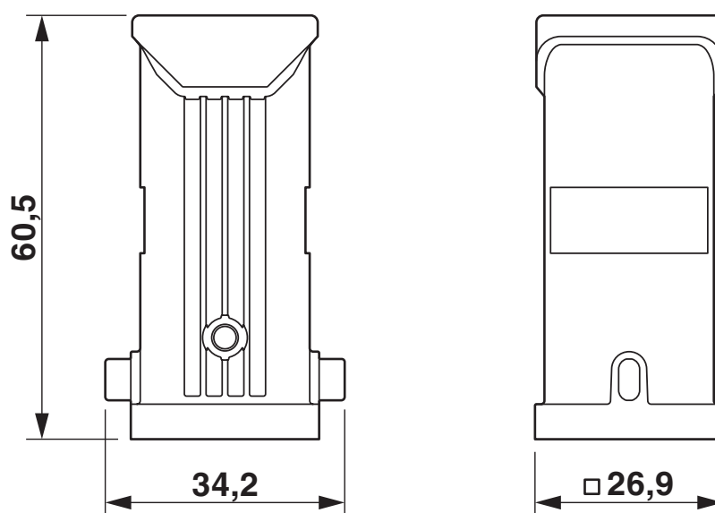
Maßzeichnung
