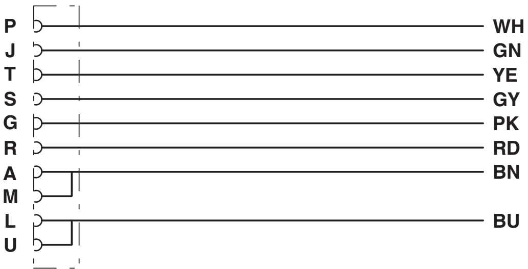
Diagrama eléctrico
