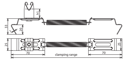
Maßbild DLH SG 8 H32 FG180.280 CU
