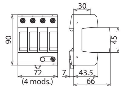
Maßbild DG MU 3PY 600 4W+G
