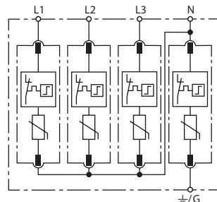
Prinzipschaltbild DG MU 3PY 600 4W+G
