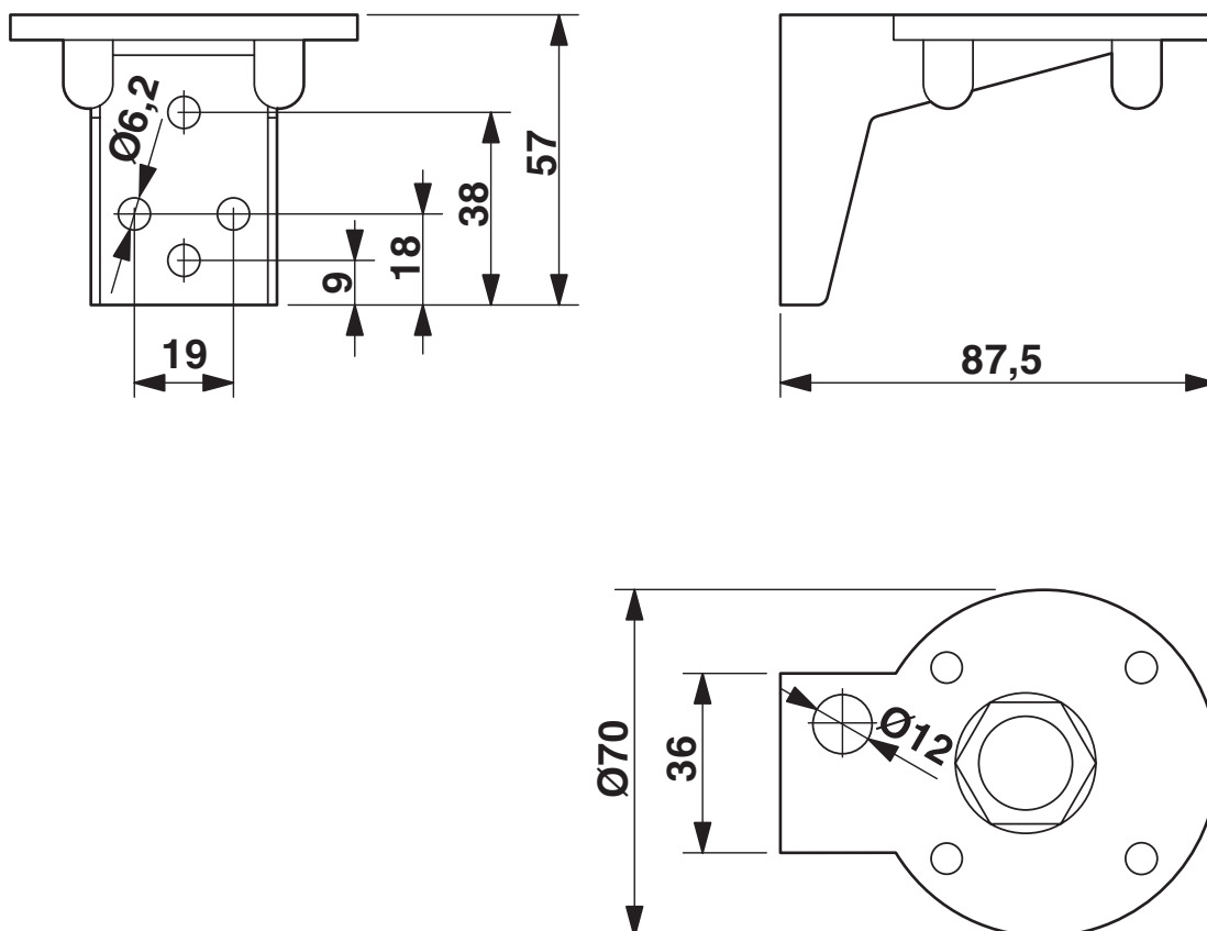
Maßzeichnung
