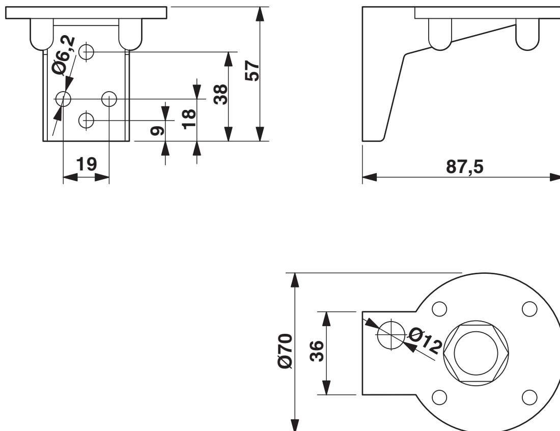
Dessin coté
