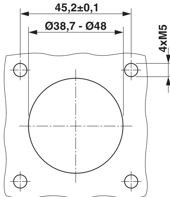
Bohrplan/Lötpadgeometrie
