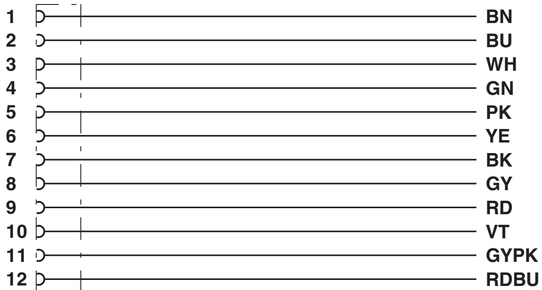
Schaltplan
